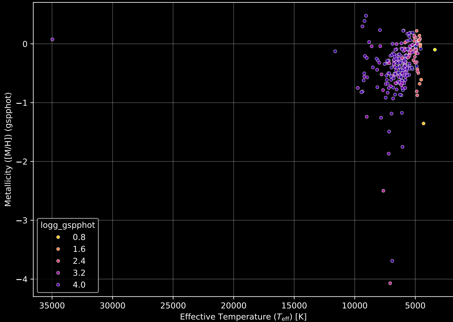
GALAH DR4 Field: [8615] Stellar Population Parameters (n= 248)
