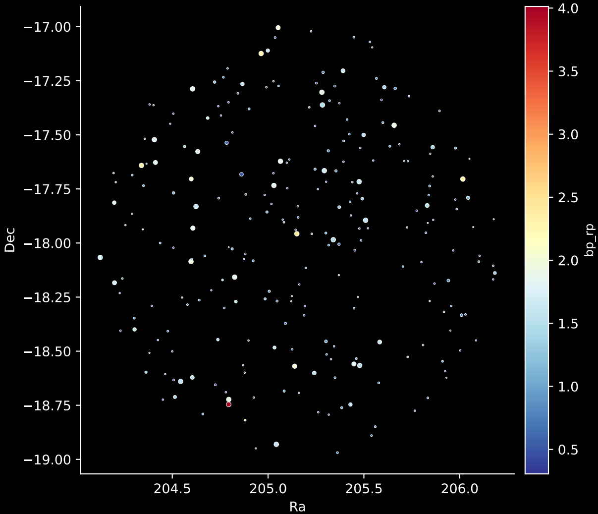
GALAH DR4 Field: [8615] Stars: 248
