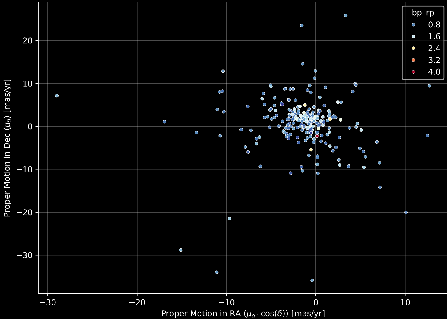
GALAH DR4 Field: [8615] Proper Motion Diagram (n= 248)
