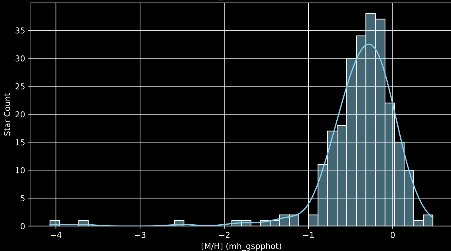
GALAH DR4 Field: [8615] [M/H] (mh_gspphot) (n= 248)
