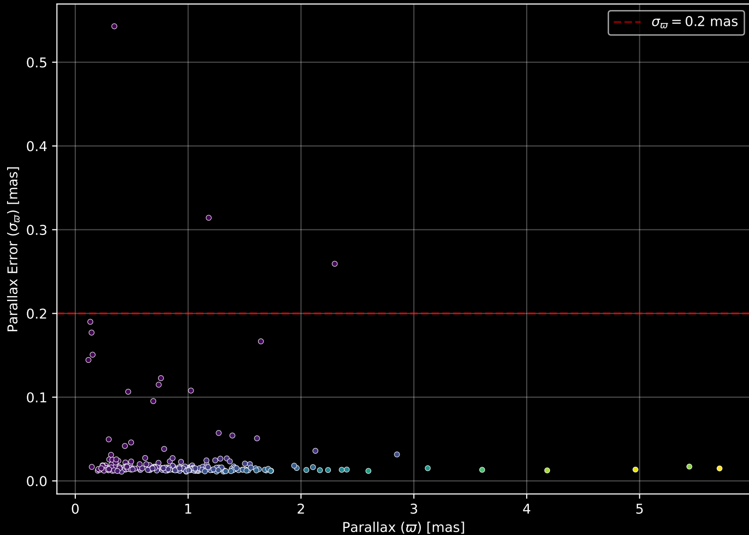
GALAH DR4 Field: [8615] Parallax Quality (n= 248)
